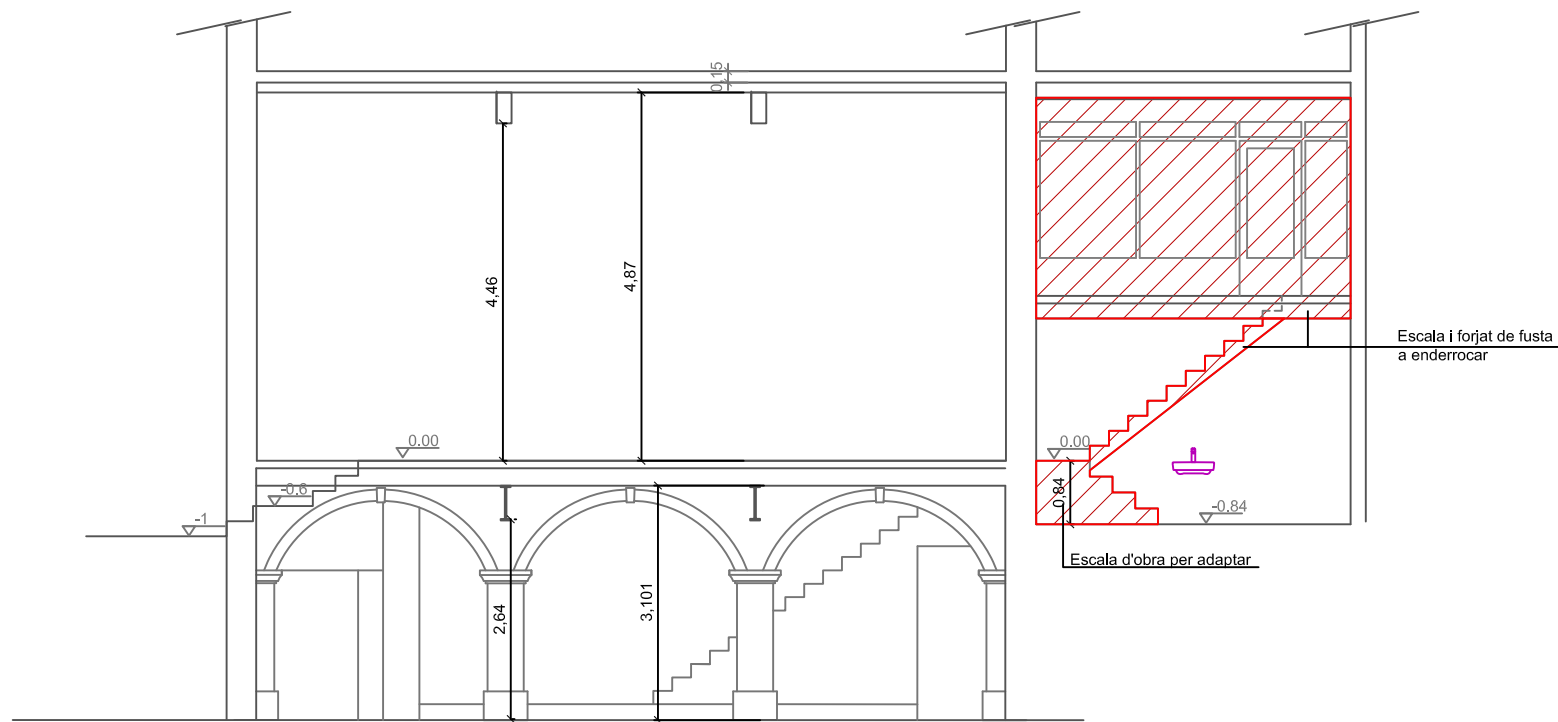
Secció A-A'
