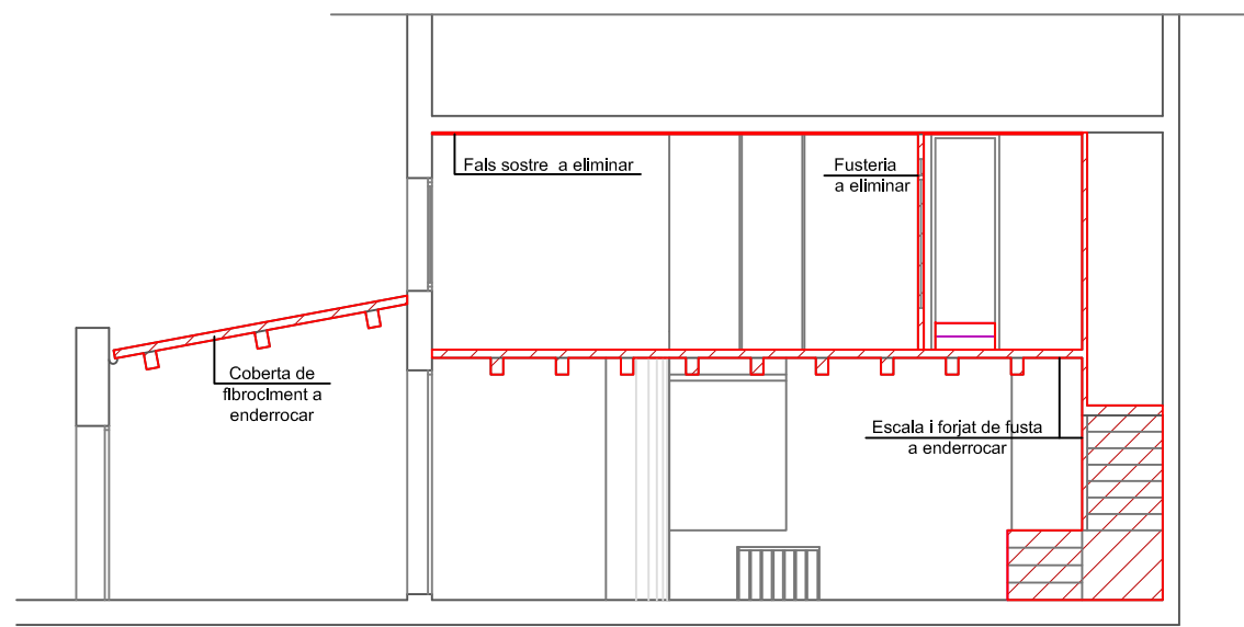
Secció B-B'
