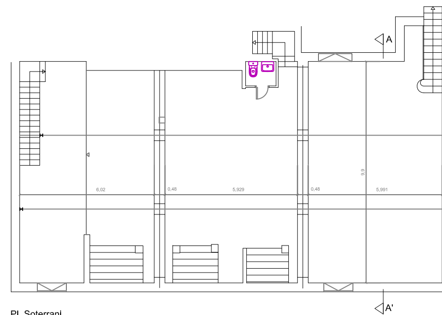
Pl. Soterrani sup. útil: 183 m2 sup. útil TOTAL pb+soterrani: 287 m2
